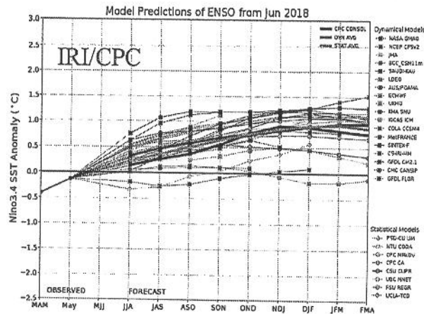
Figura 2. Pluma de Pronóstico del fenómeno El Niño Agosto-Septiembre-October, año 2018.
