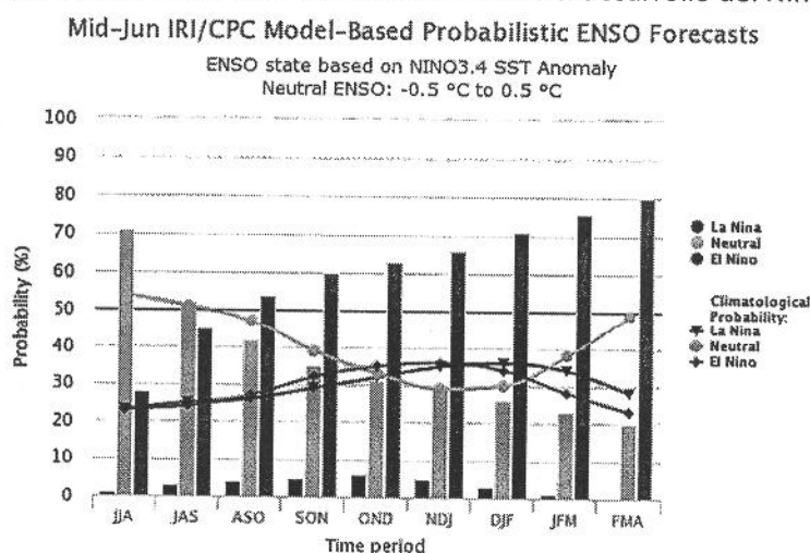
Figura 1. Probabilidad de ocurrencia del fenómeno El Niño Julio-Agosto-Septiembre, año 2018.
