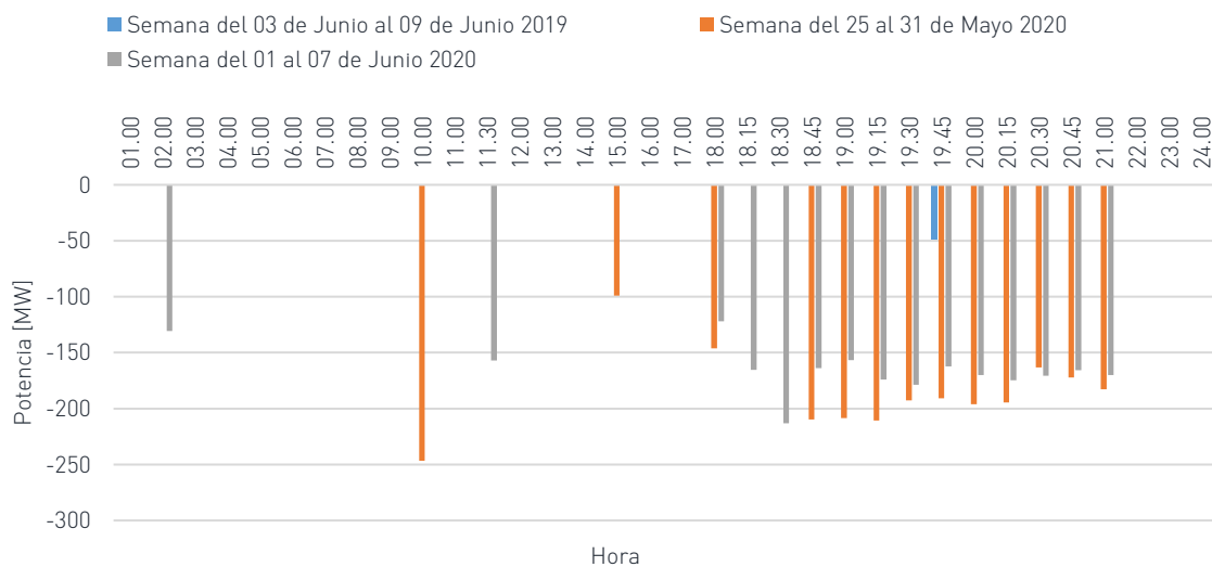
Gráfica 20: Balance de la potencia semanal promedio.
