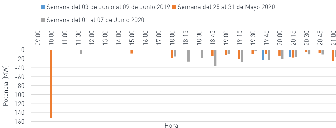
Gráfica 12: Potencia semanal promedio importada del MER.
