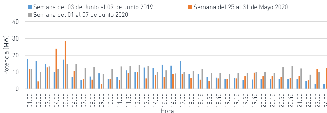
Gráfica 8: Potencia semanal promedio suministrada por plantas Eólicas del S.N.I.
