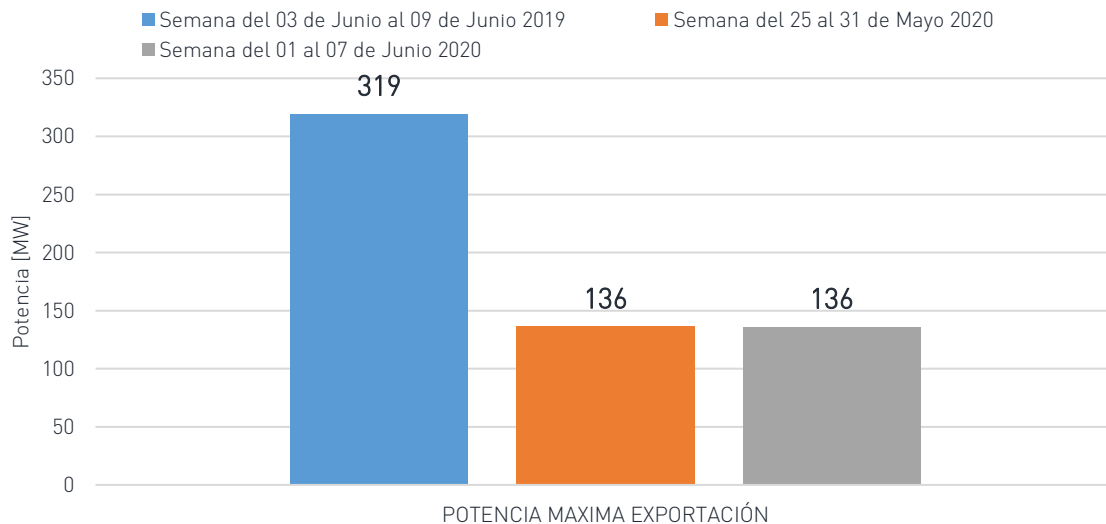
Gráfica 11: Potencia máxima Exportada al MER.
