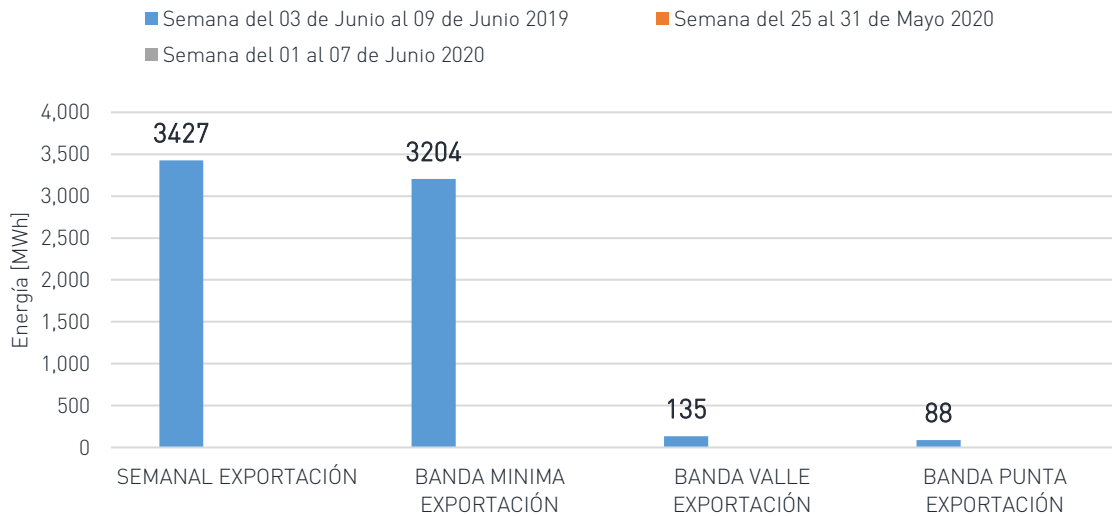
Gráfica 15: Energía semanal exportada a MEX.
