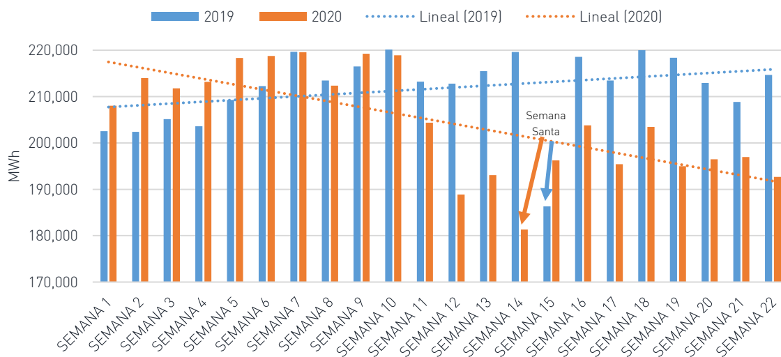
Gráfica 2: Demanda de Energía Eléctrica semanal.
