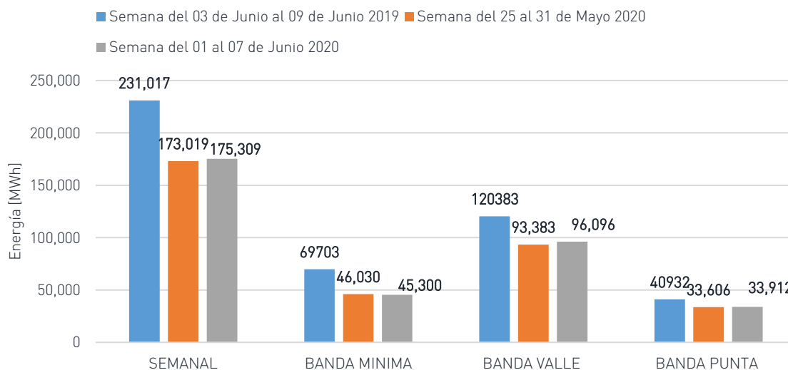
Gráfica 5: Comparación la energía semanal Generada.
