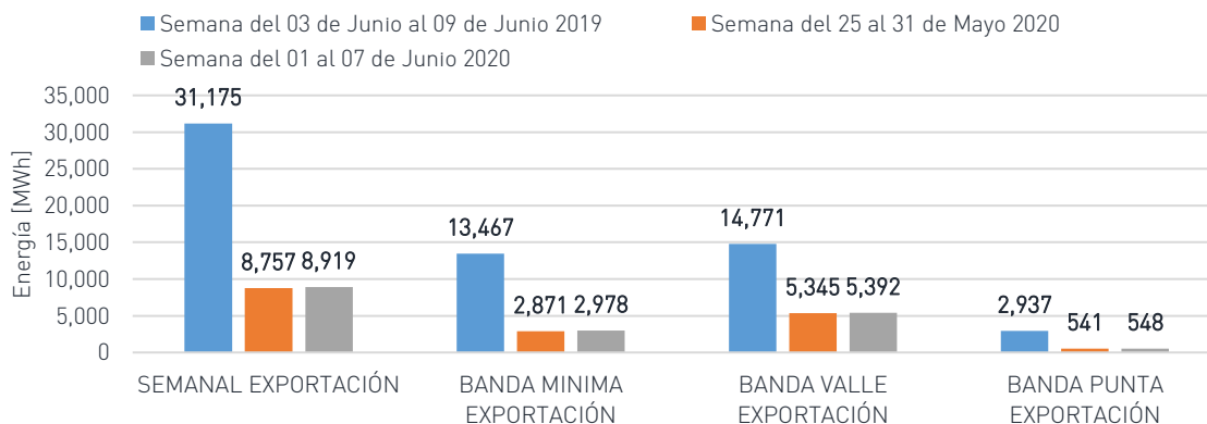
Gráfica 10: Energía semanal Exportada al MER.
