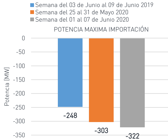
Gráfica 19: Potencia máxima importada de MEX.
