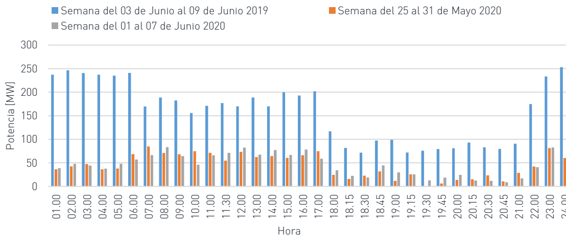
Gráfica 9: Potencia semanal promedio exportada al MER.
