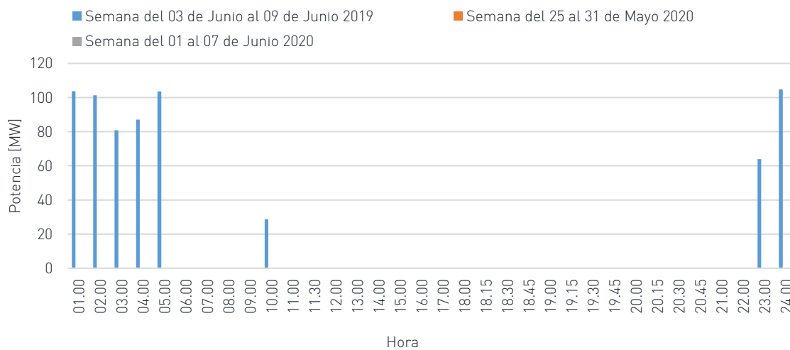
Gráfica 14: Potencia semanal promedio exportada a MEX.
