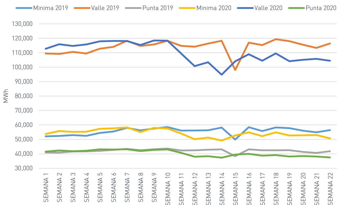
Gráfica 3: Demanda de Energía Eléctrica semanal.
