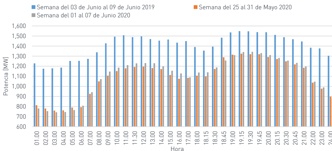
Gráfica 4: Comparación de potencia semanal generada.
