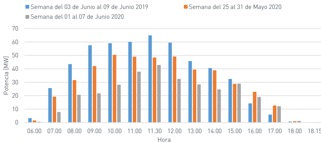
Gráfica 7: Potencia semanal promedio suministrada por plantas solares del S.N.I.
