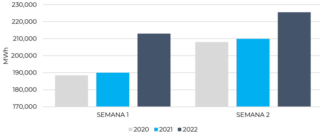
Demanda de energía semanal del SNI 2020, 2021 y 2022
