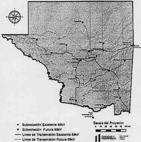
RED DE TRANSMISIÓN ACTUAL 69KV Y CON EL PET 2022 - 2052 DEL DEPARTAMENTO DE PETÉN
