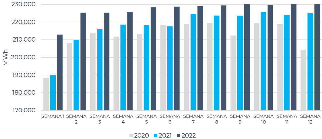
Demanda de energía semanal del SNI 2020, 2021 y 2022
