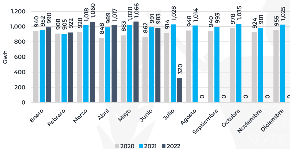
Demanda de energía mensual del SNI
