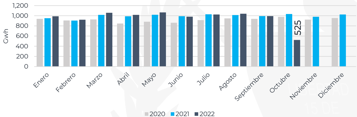
Demanda de energía mensual del SNI
