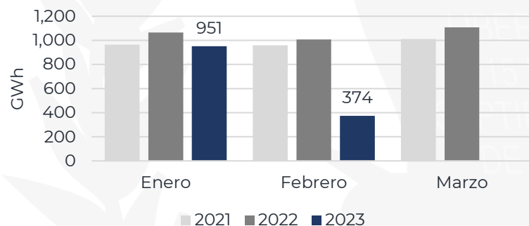
Gráfica 5: Generación Mensual S.N.I
