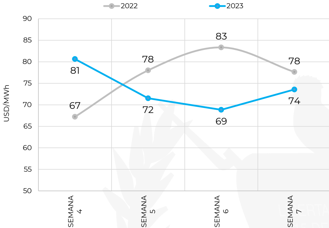
Gráfica 6: Costo semanal promedio SPOT.
