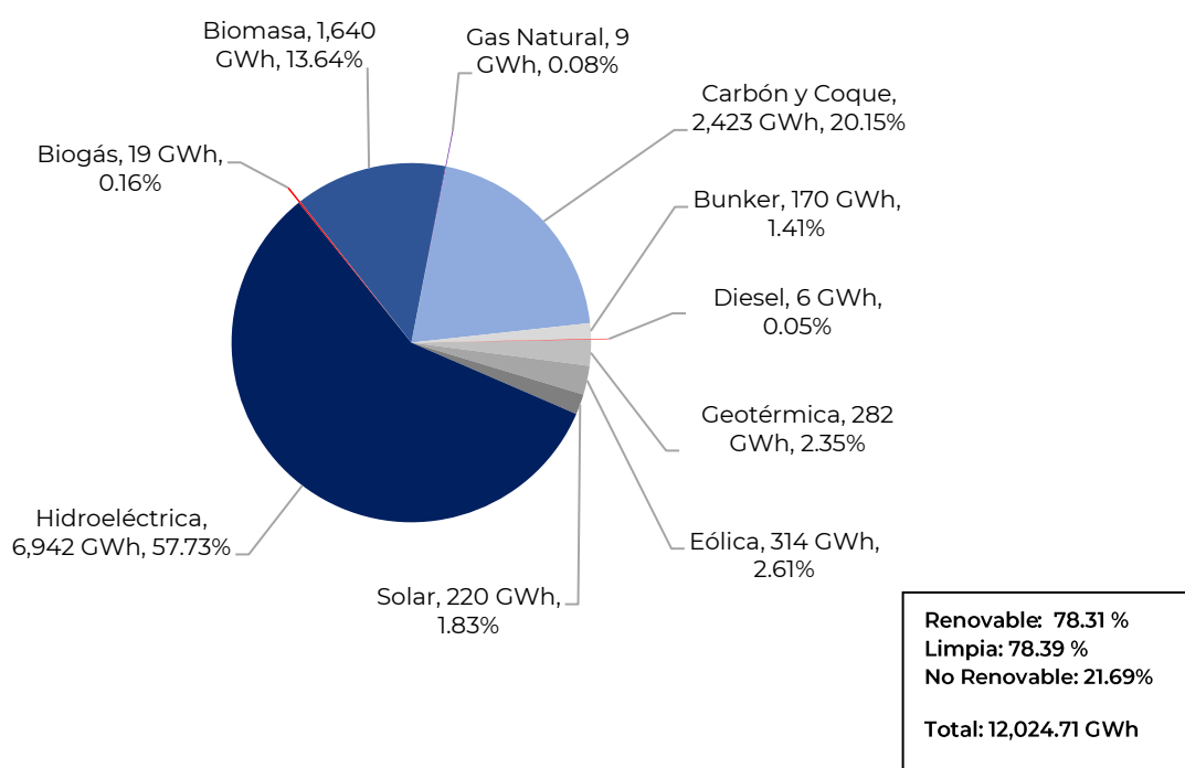
Gráfica 16: Matriz Energética Por Tipo de Tecnología 2022.
