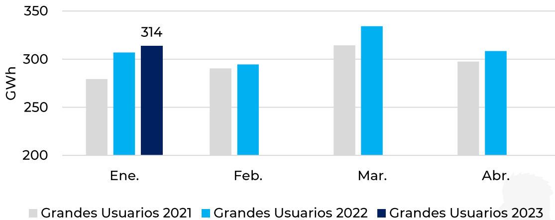
Gráfica 12: Demanda de Energía Mensual G.U.
