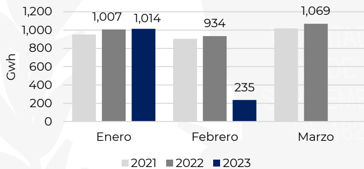
Gráfica 2: Demanda de energía mensual del S.N.I.
