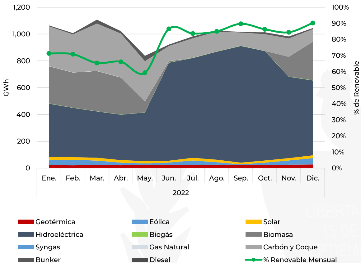
Gráfica 14: Generación por Tipo de Recurso en el SNI.
