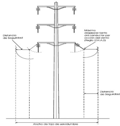
Figura 1: Faja de servidumbre
