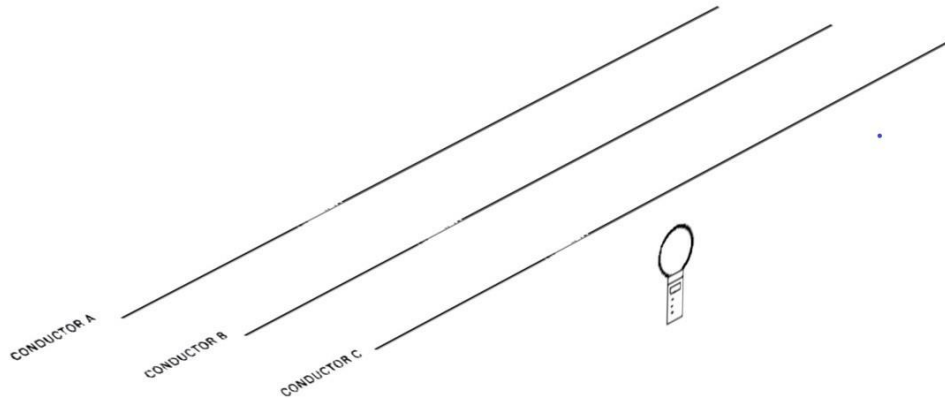
Figura 3: Orientación de la sonda para realizar la medición del campo magnético.
