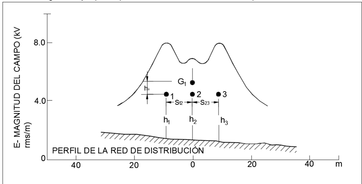
Figura 6: Ejemplo de perfil lateral de la intensidad del campo eléctrico
