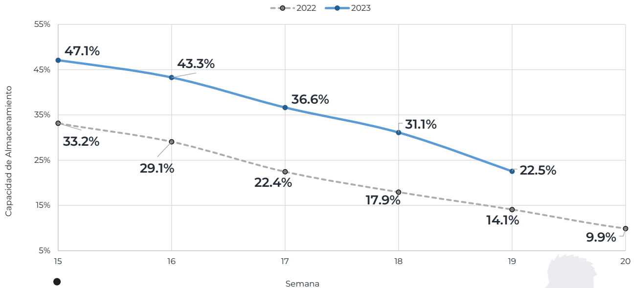
Gráfica 6. Porcentaje de Almacenamiento Efectivo del Embalse CHIXOY.
