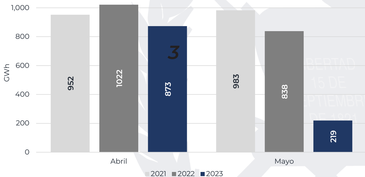
Gráfica 5. Generación Mensual S.N.I
