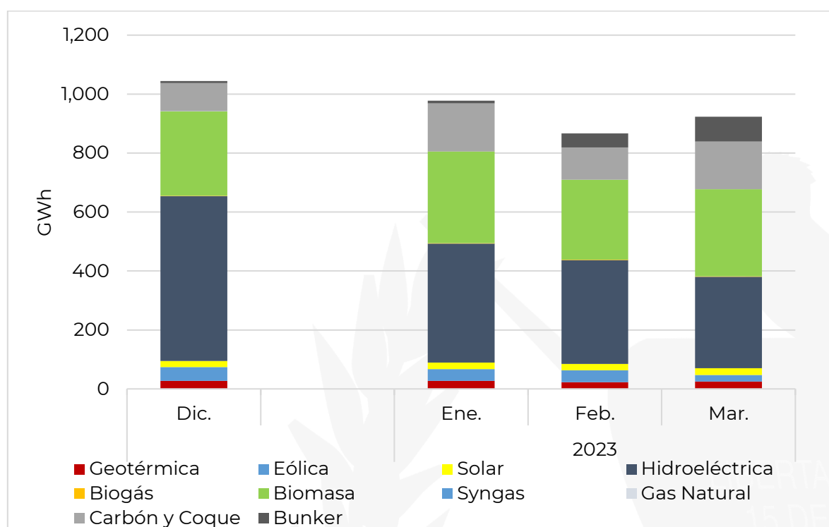
Gráfica 14: Generación por Tipo de Recurso en el SNI.
