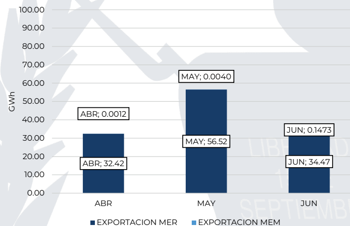
Gráfica 18. Exportaciones S.N.I.
