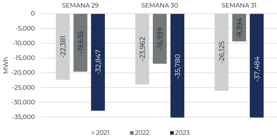
Gráfica 8. Intercambios de Energía Netos por Semana en Interconexión con México .
