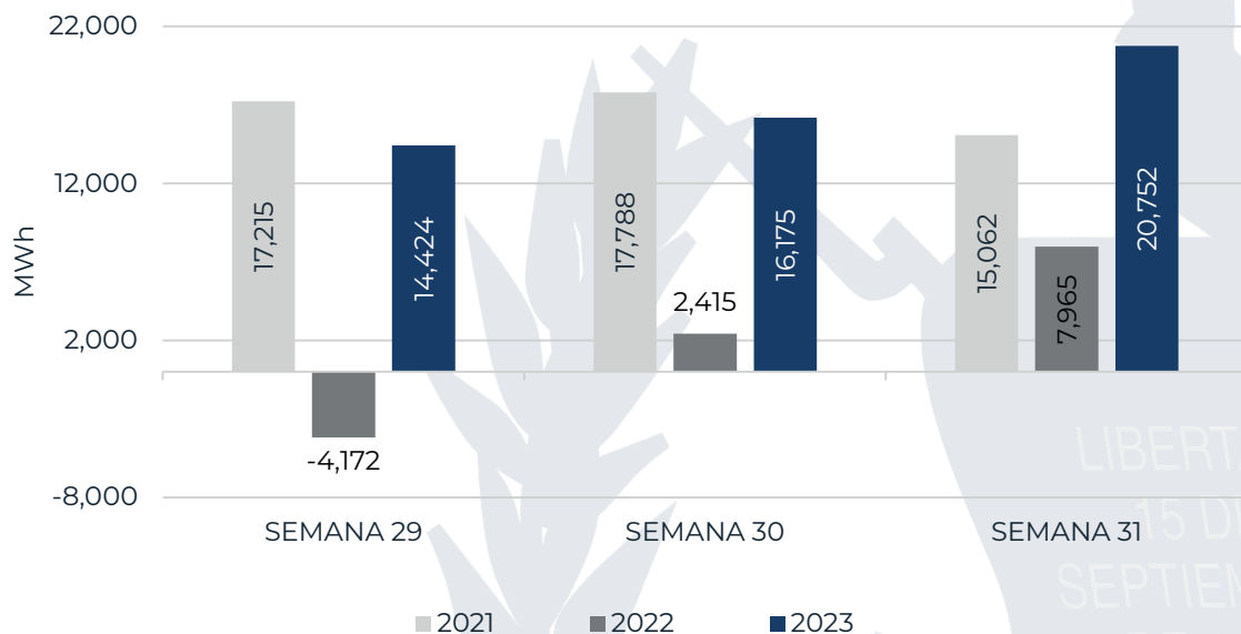
Gráfica 9. Intercambios de Energía Netos por Semana con el Mercado Eléctrico Regional.
