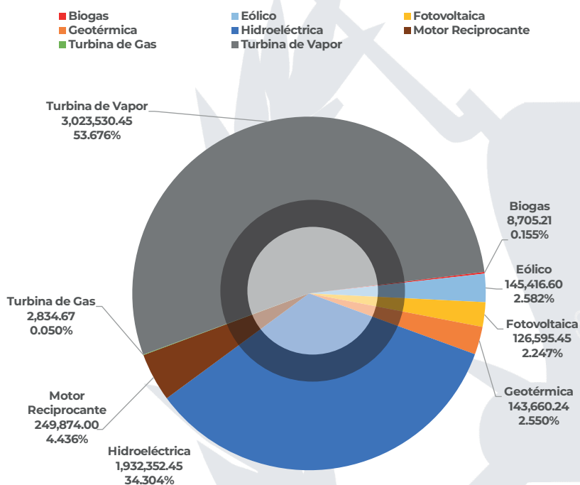
Gráfica 16. Matriz Energética Por Tipo de Tecnología.
