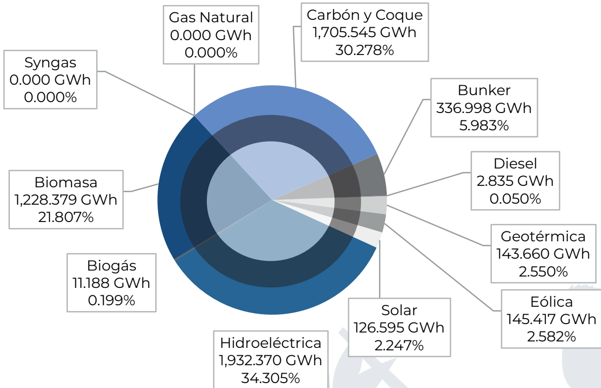
Gráfica 14. Matriz Energética Por Tipo de combustible.
