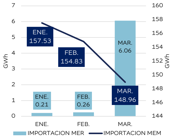
Gráfica 19. Importaciones mensuales al SNI
