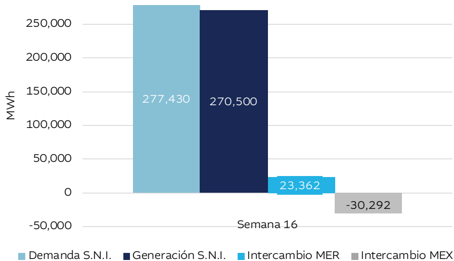
Gráfica 1. Balance Eléctrico Semanal
