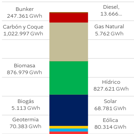
Gráfica 16. Generación por tipo de recurso en el SNI
