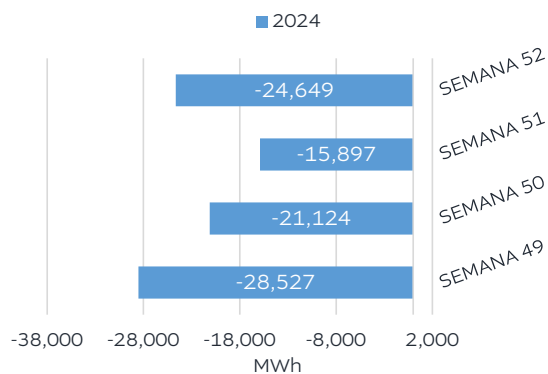
Gráfica 9. Intercambios semanales de energía netos en Interconexión con Mercado Eléctrico Mexicano
