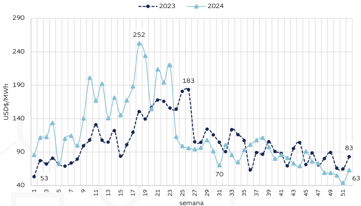
Gráfica 11. Promedio semanal del Precio Spot de energía eléctrica
