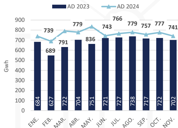
Gráfica 15. Evolución de la demanda mensual de Agentes Distribuidores
