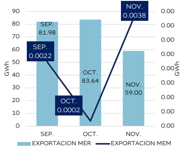
Gráfica 20. Exportaciones mensuales del SNI
