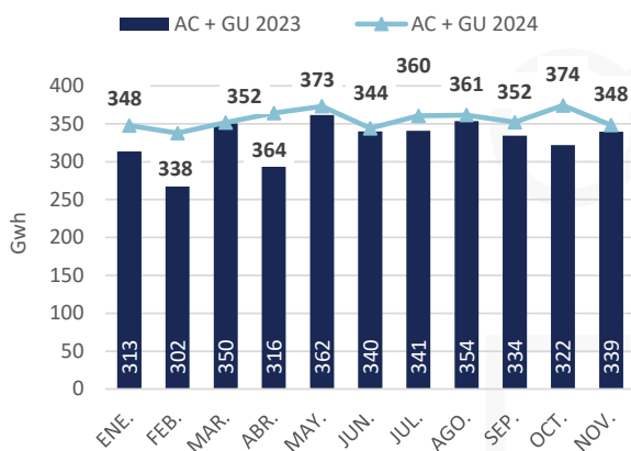
Gráfica 14. Evolución de la demanda mensual de Comercializadores y Grandes Usuarios
