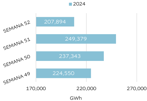
Gráfica 5. Generación de energía semanal del SNI
